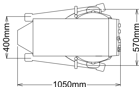
Boven aanzicht
