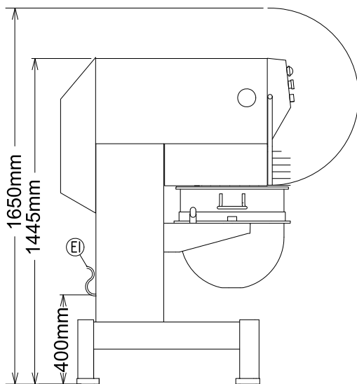
Zij aanzicht
